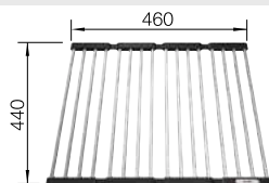
KlappMatte - sklopná mřížka multifunkční mřížka 460x440 mm
