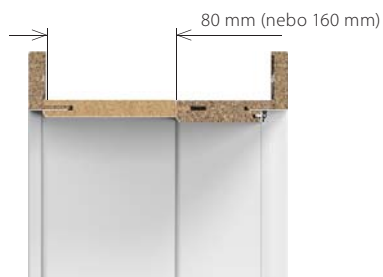
verze s regulačním panelem (80, 160 mm)
