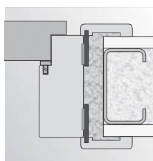
montáž do pěny do stěny ze sádkartonové desky
