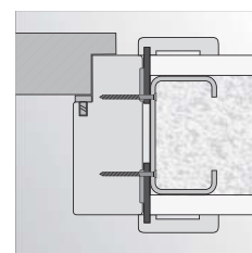
montáž na vruty do stěny ze sádkartonové desky
