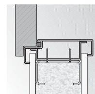
rohová zárubeň velká montáž do sádkartonové stěny
