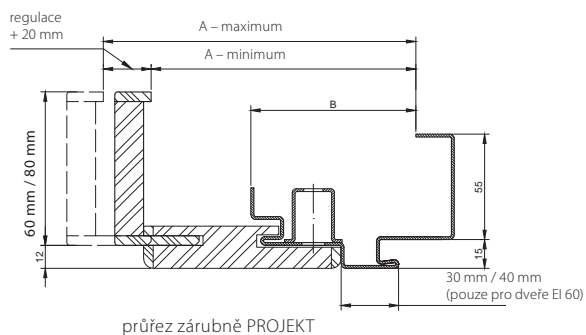
průřez zárubně PROJEKT
