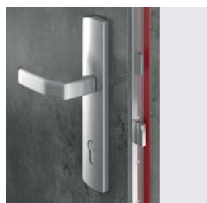
lištový zámek Winkhaus vícebodový hákové-zásuvkový
