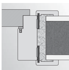
montáž do pěny do zděné stěny
