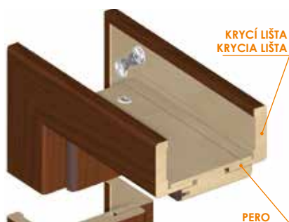
ORS1 ÚHELNÍK S PLOCHOU KRYCÍ LIŠTOU O ŠÍŘCE 60 MM A PEREM 30 MM (STANDARD) ROHOVNÍK S PLOCHOU KRYCOU LIŠTOU SO ŠÍRKOU 60 MM A PEROM 30 MM (STANDARD)
