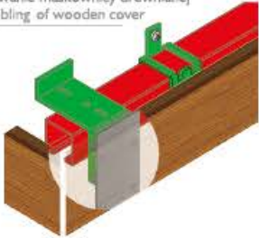
mocowanie maskownicy drewnianej assembling of wooden cover
