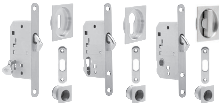
Zestaw na klucz BB
