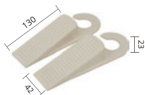
Stoper 2080 klin (2 szt.)
