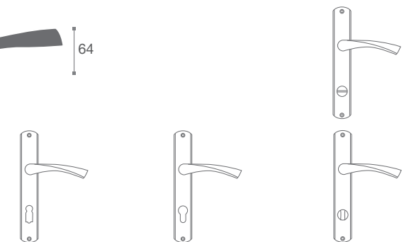
Panino BB Panino PZ Panino WC 248322 248323 248333
