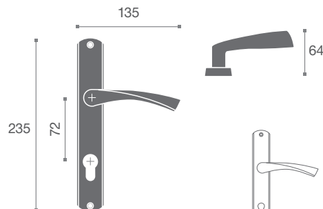
Panino BB Panino PZ Panino WC 248322 248323 248333
